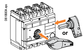
Стандартная поворотная рукоятка: INS250 и INV100 - 250
