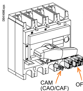
Compact INS/INV320 - 630
