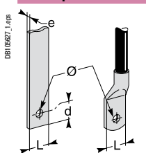
Присоединение шин или кабелей с наконечниками
